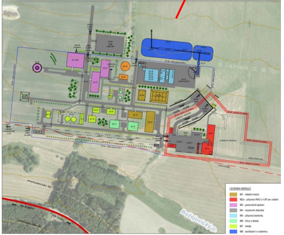
Dispoziční řešení D2 - vertikální ukládání, konvenční ražba
