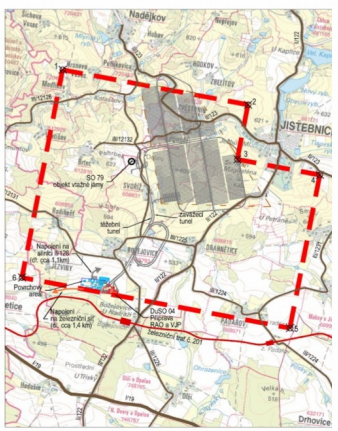
Dispoziční řešení D3 - horizontální ukládání, ražba TBM
