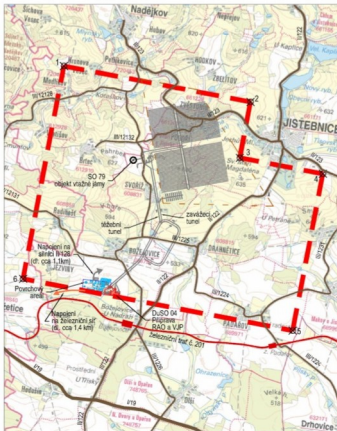
Dispoziční řešení D2 - vertikální ukládání, konvenční ražba
