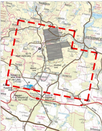
Dispoziční řešení D1 - vertikální ukládání, ražba TBM
