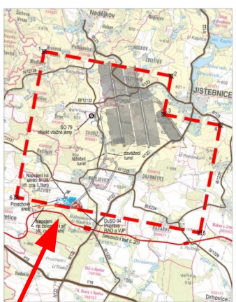
Dispoziční řešení D4 - horizontální ukládání, konvenční ražba
